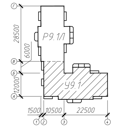
Схема компоновки
