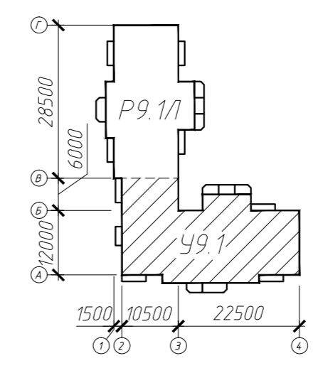
Схема компоновки
