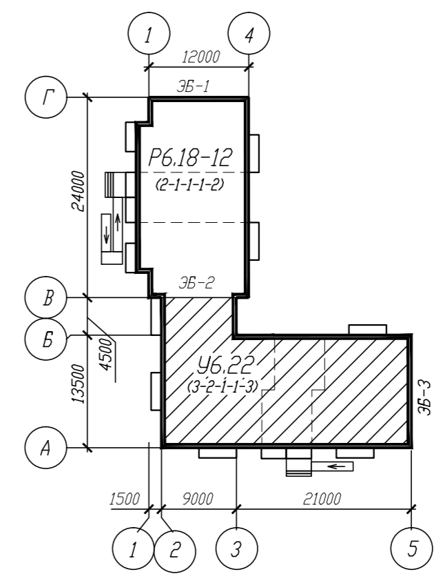
Схема компоновки
