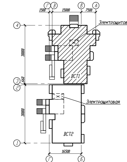
Схема компоновки
