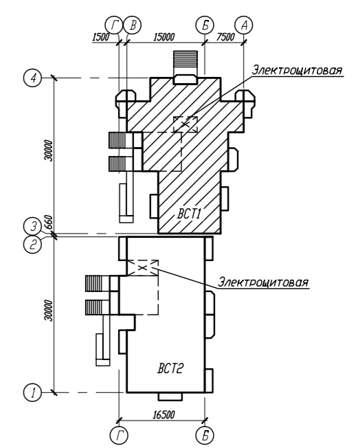
Схема компоновки
