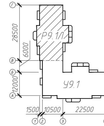
Схема компоновки
