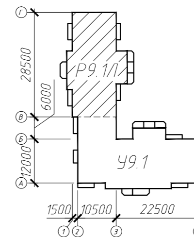
Схема компоновки
