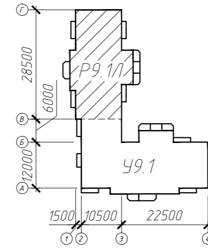
Схема компоновки
