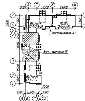
Схема компоновки
