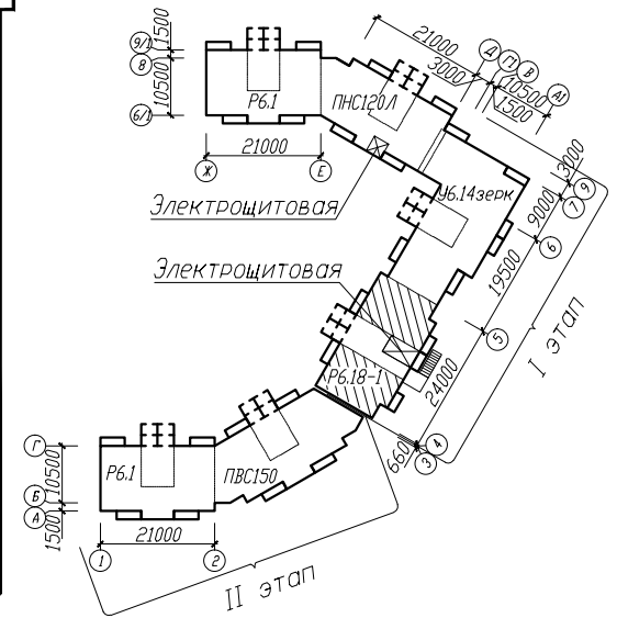
СХЕМА КОМПОНОВКИ
