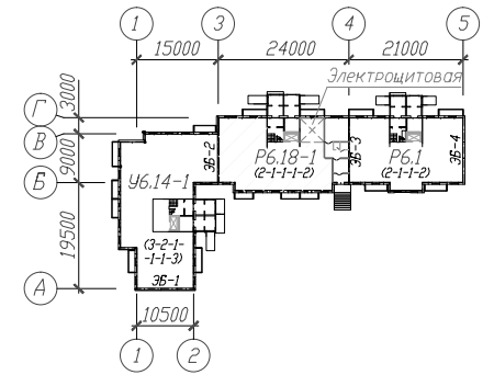
СХЕМА КОМПОНОВКИ
