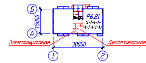
СХЕМА КОМПОНОВКИ
