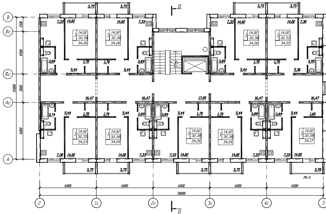
СХЕМА КОМПАКОВКИ
