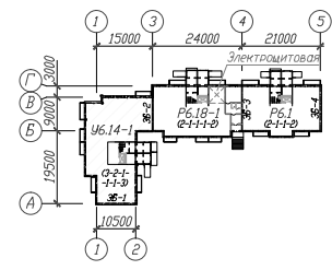
СХЕМА КОМПОНОВКИ
